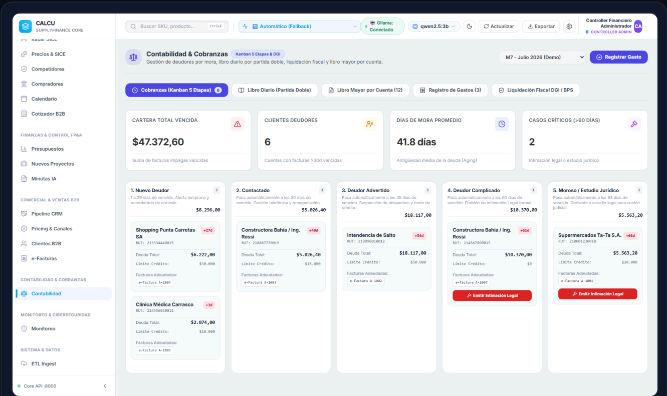
Figura 6.1: Tablero Kanban de Cobranzas en 5 etapas con cálculo de días de atraso y límite de crédito. Módulo: Contabilidad / Cobranzas
