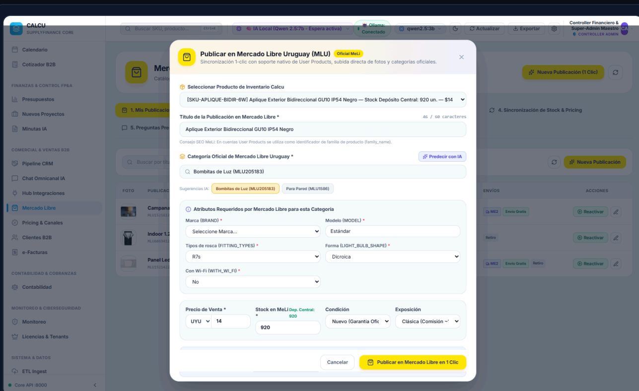
Figura 24.1: Modal de Publicación Asistida en Mercado Libre Uruguay con predicción semántica de categoría y formulario dinámico de atributos obligatorios.
