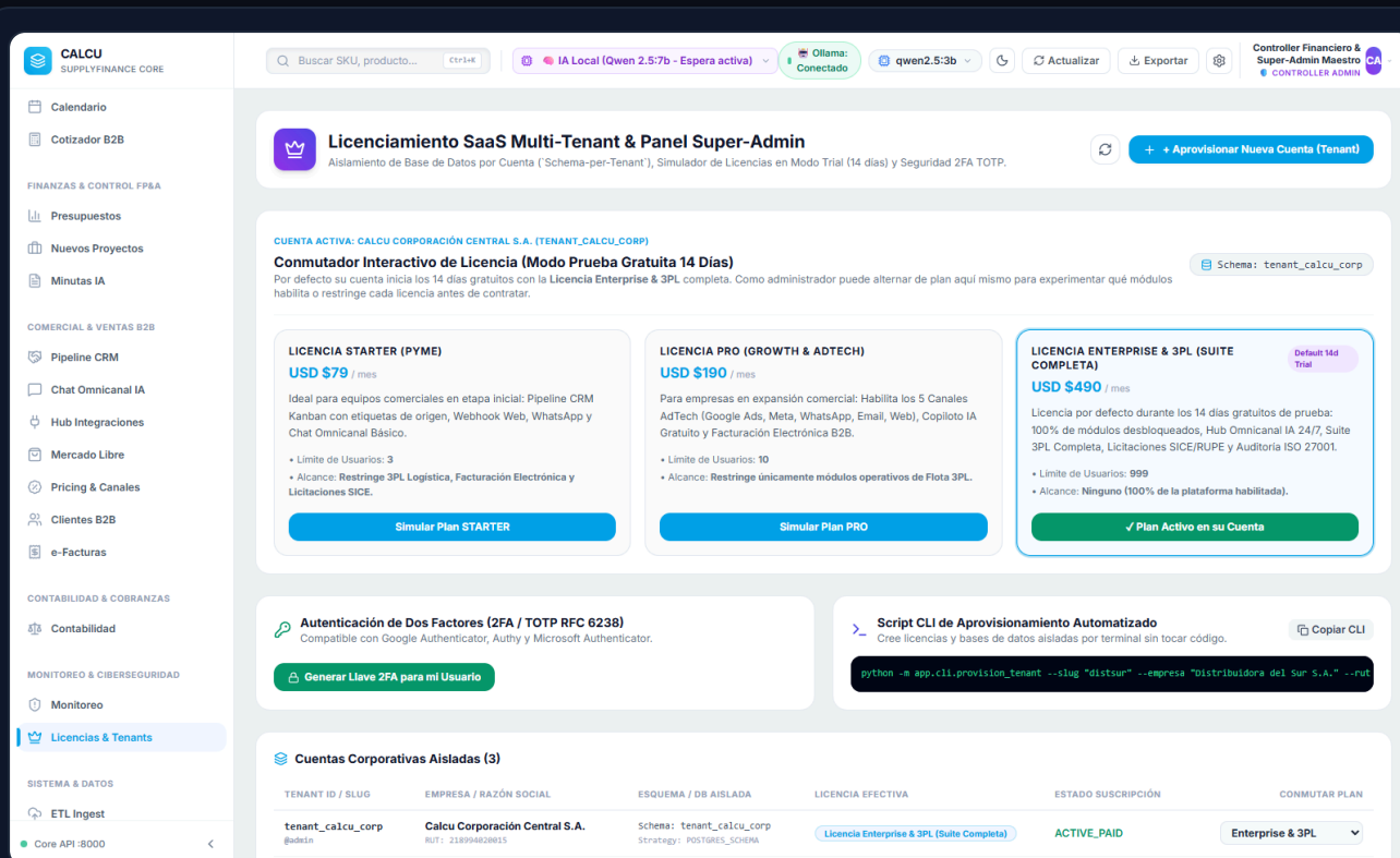
Figura 25.1: Panel Super-Admin de Licenciamiento SaaS con simulador de planes en modo prueba, aprovisionamiento automatizado y seguridad 2FA TOTP. Módulo: Monitoreo & Ciberseguridad / Licencias & Tenants
